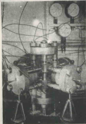
Рис. 2. Общий вид шестикомпонентной установки
